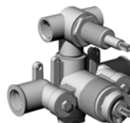
Ref. M00-2T24 Centrale thermostatique avec 1 robinet d'arrêt-inverseur 2 sorties (55 l/mn) Thermostatic mixer with a 2 ways diverter on-off (55l/mn)
